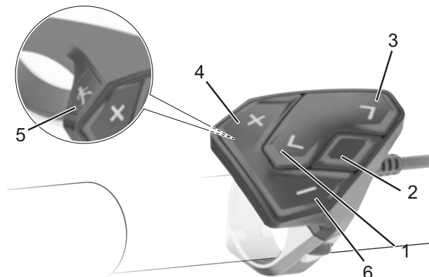
Figura 22: Schema del terminale di comando
