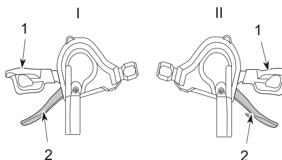
Figura 83: Leva del cambio al rapporto minore (1) e leva del cambio al rapporto maggiore (2) del cambio sinistro (I) e destro (II)
