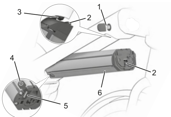
Figura 18: Dettaglio della batteria integrata
