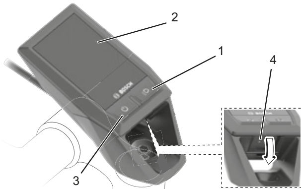
Figura 19: Schema della struttura e degli elementi di comando del display
