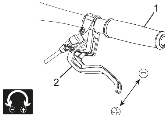
Figura 56: Uso della vite di regolazione (2) per regolare la distanza della leva del freno dalla manopola del manubrio (1)
