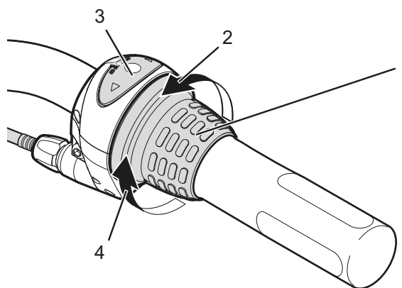
Figura 84: Esempio: cambio Shimano Nexus: interruttore a manopola (1) del cambio al mozzo con display (3), senso di rotazione per passare al rapporto superiore (2) e senso di rotazione per passare al rapporto inferiore (4)
