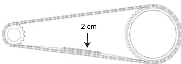
Figura 85: Controllo della tensione della catena
