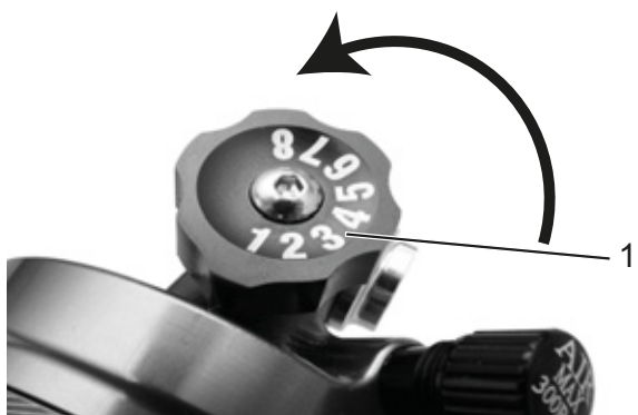
Figura 63: Regolatore della compressione Suntour sull'ammortizzatore del carro posteriore
