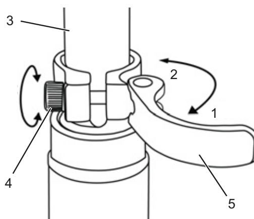
Figura 48: Bloccaggio rapido del canotto reggisella (3)
