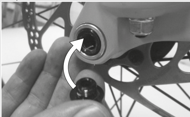
Figura 28: Applicazione della leva del bloccaggio rapido nel perno
