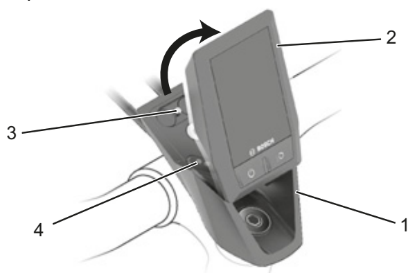
Figura 72: Sbloccare il display (2) dal supporto (1) con la vite di bloccaggio (3) del display e allontanarlo dai contatti.
