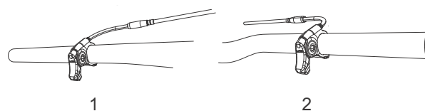
Figura 50: La leva di azionamento del canotto reggisella può essere montata a sinistra (1) o a destra (2) sul manubrio
