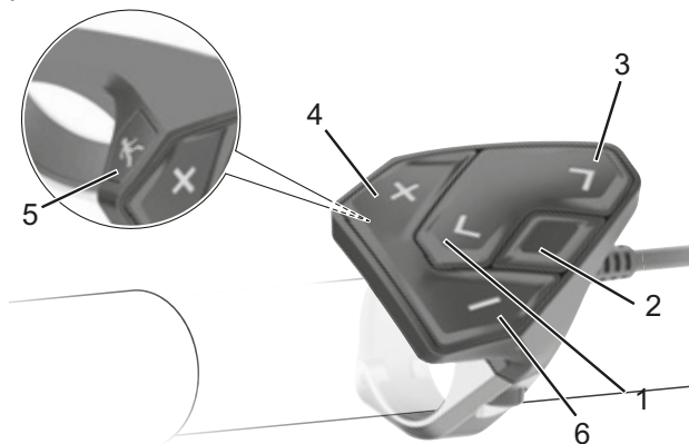
Figura 73: Schema del terminale di comando
