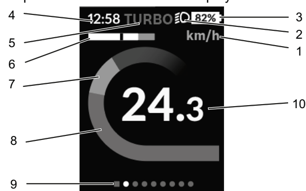
Figura 23: Schema della pagina iniziale
